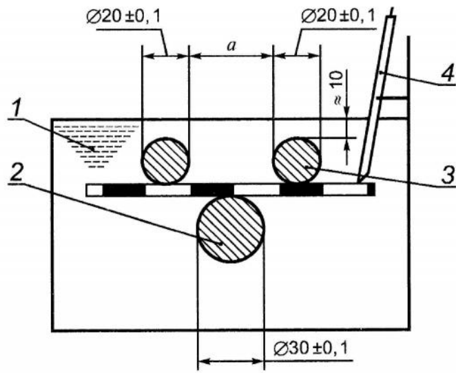
а) Начало изгибания
