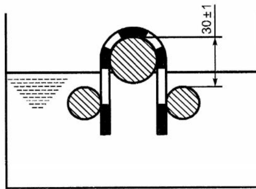
б) Конец изгибания
