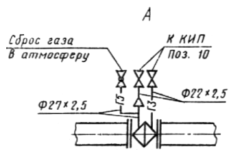
Схема ГРУ
