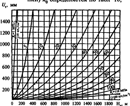
Рис. 1. Графики для определения типового смещения пород U_T
