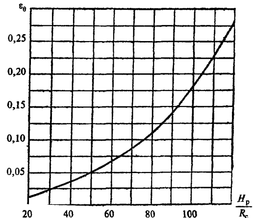
Рис. 3. График для определения \epsilon_0
