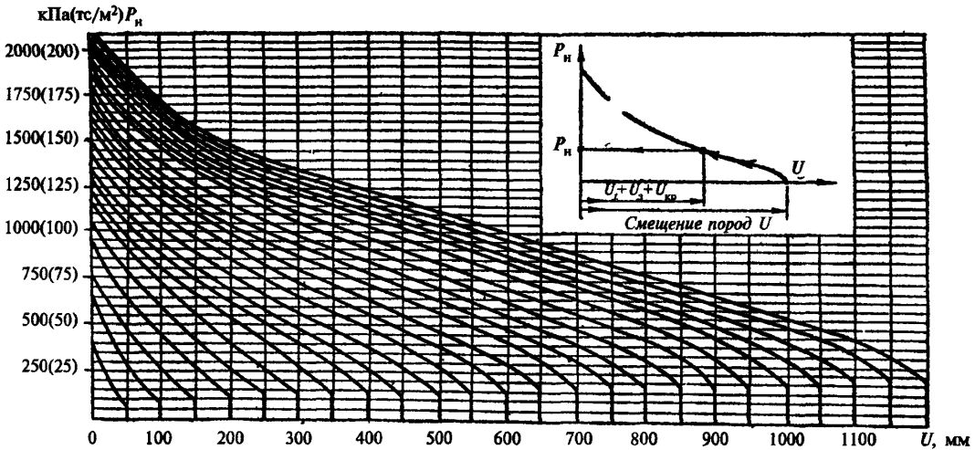
Рис. 4. Графики для определения нормативной нагрузки на крепь
