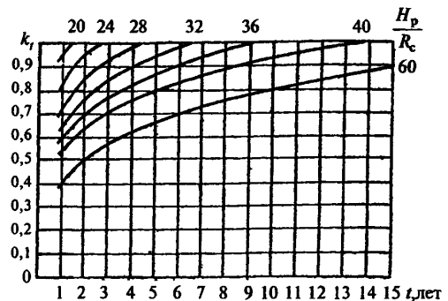
Рис. 2. Графики для определения коэффициента k_t при t от 1 года до 15 лет
