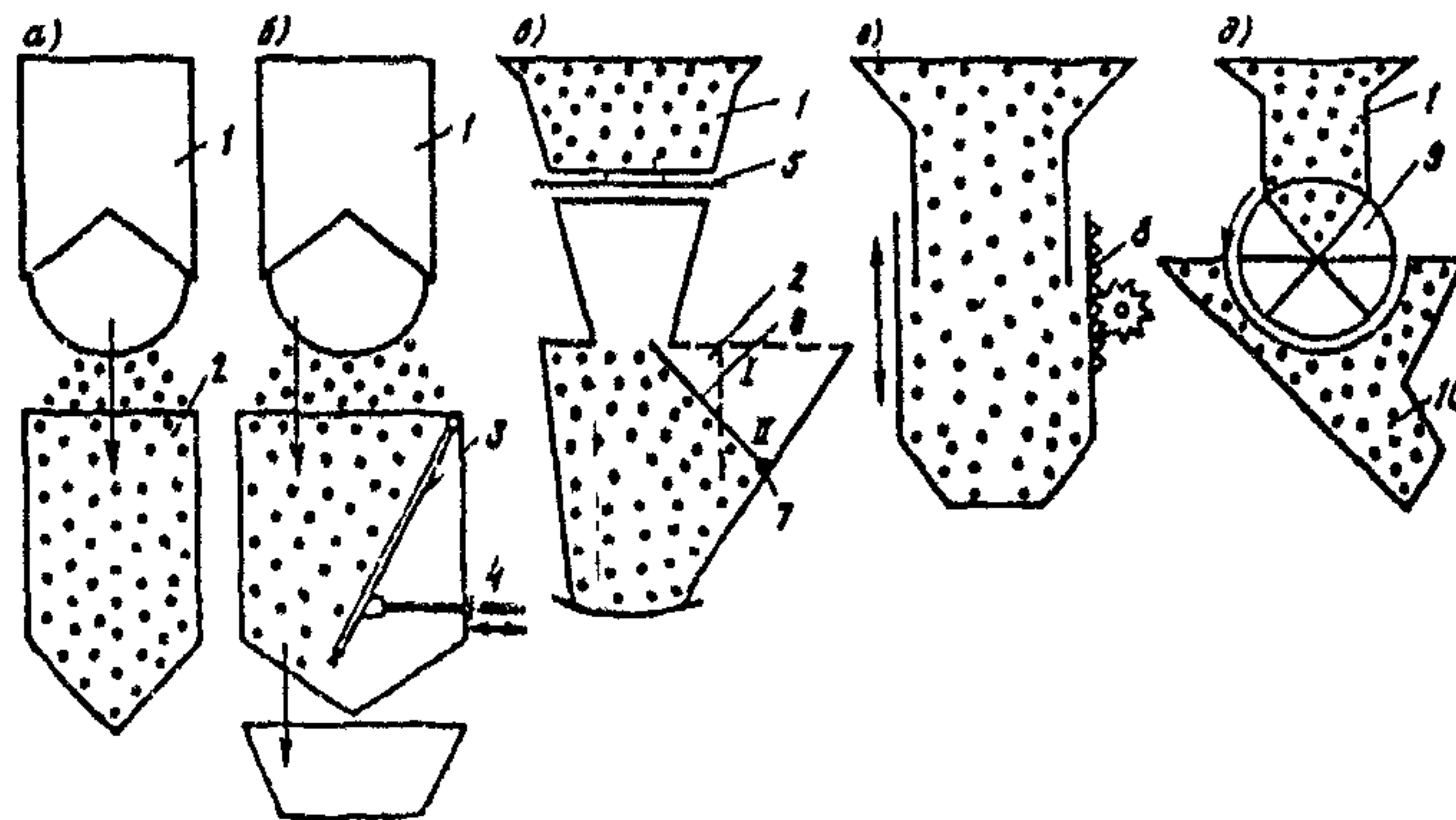
Рис. 6. СХЕМЫ ОБЪЕМНО-ВЕСОВЫХ ДОЗАТОРОВ (по данным ВНИИжелезобетон)
