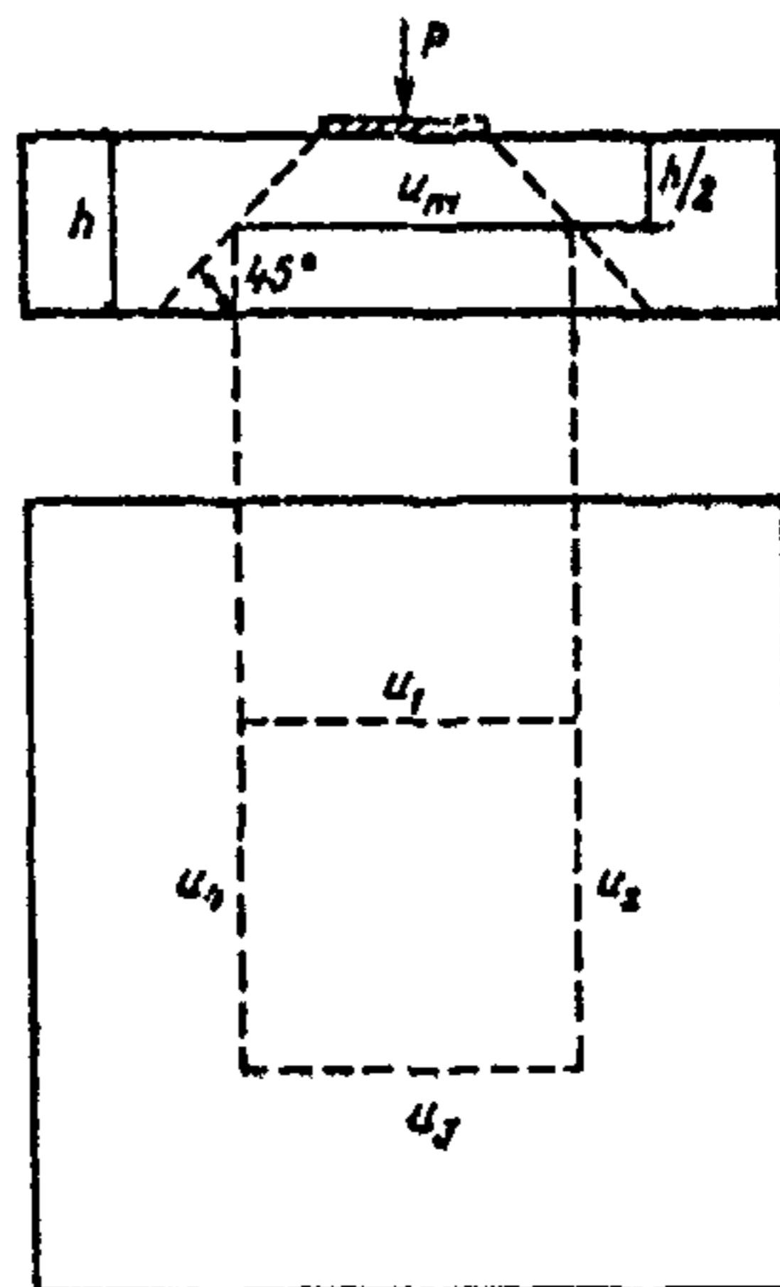
РИС. 3. СХЕМА ОБРАЗОВАНИЯ ПИРАМИДЫ ПРИ ПРОДАВЛИВАНИИ ЭЛЕМЕНТА ИЗ АРБОЛИТА
