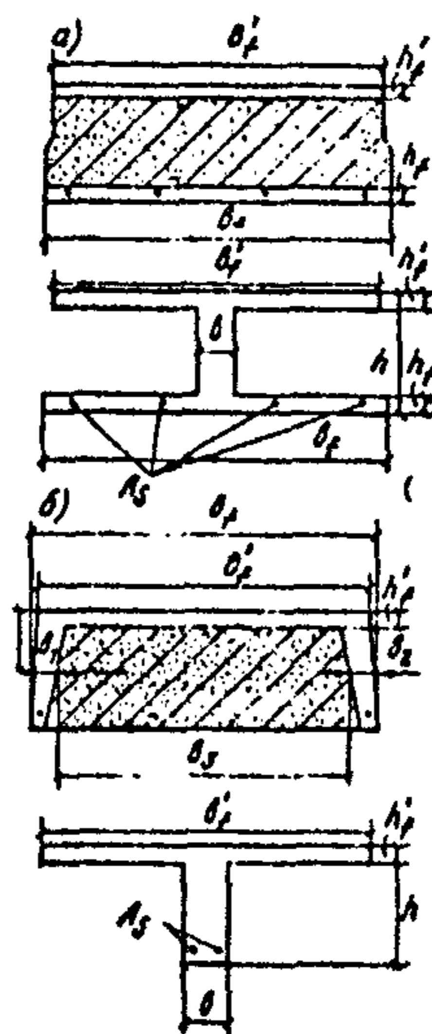
РИС. 4. СХЕМА ПОПЕРЕЧНЫХ СЕЧЕНИЙ СОСТАВНЫХ ЭЛЕМЕНТОВ
