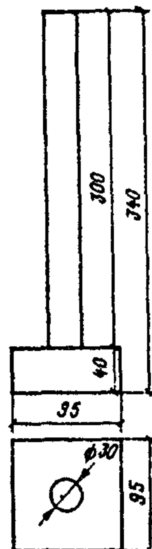
РИС. 5. СТАЛЬНАЯ БОЛВАНКА ДЛЯ ТРАМБОВАНИЯ
