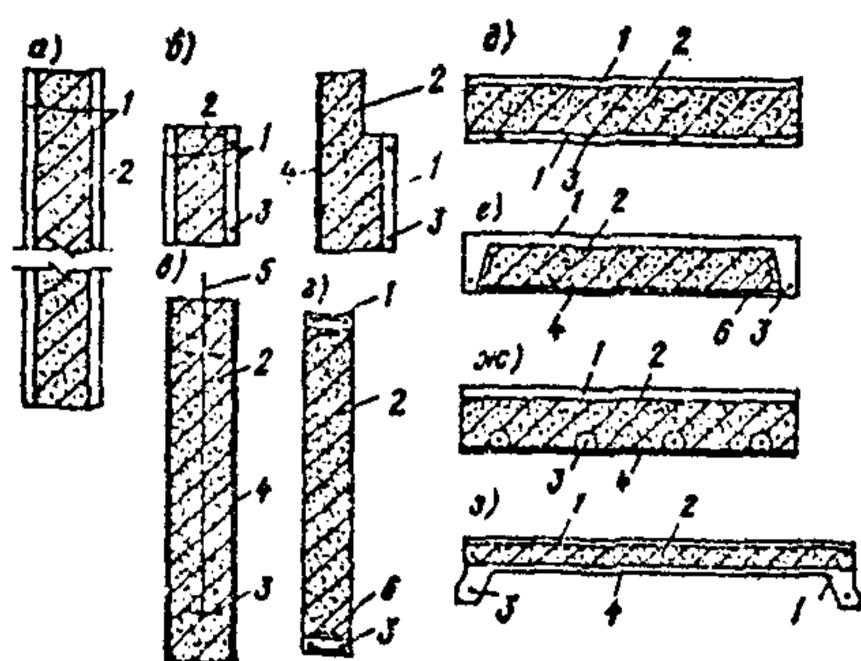
РИС. 1. ЭЛЕМЕНТЫ ИЗ АРБОЛИТА И БЕТОНА
