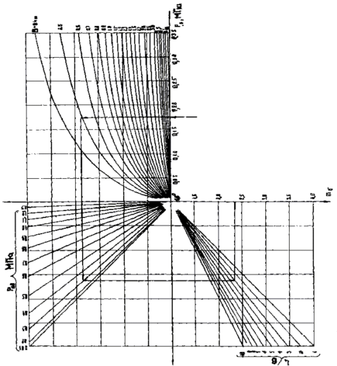
Рис. 2. Значение коэффициента m_b , учитывающего формоизменение грунта под фундаментом
