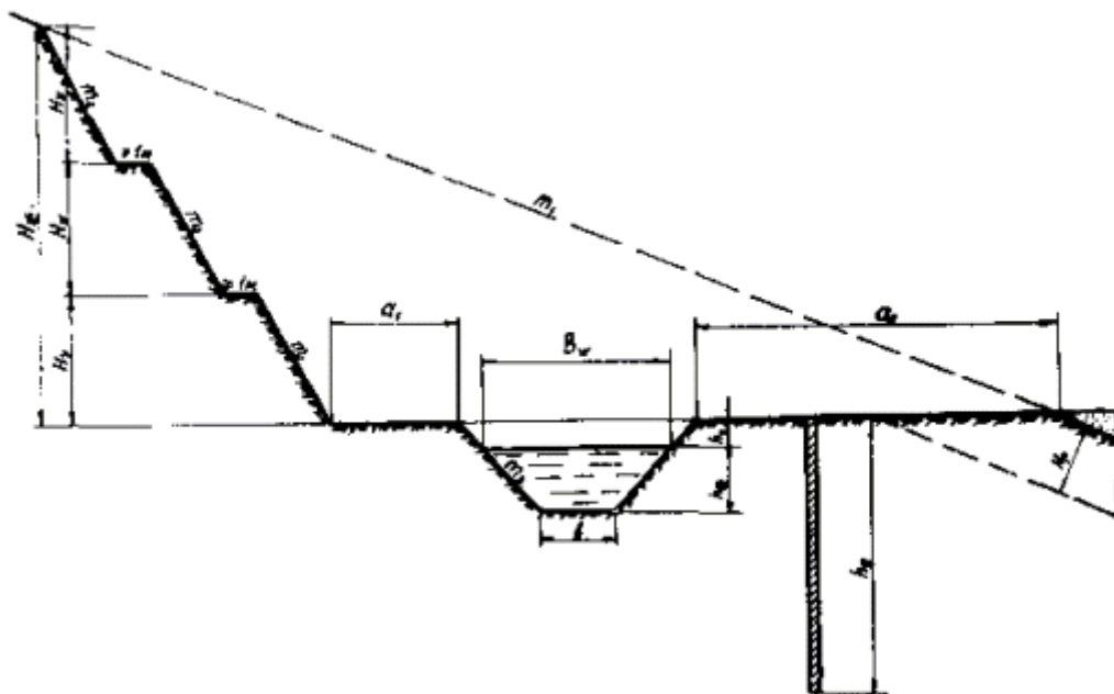
Рис. 2 Канал на косогоре.
