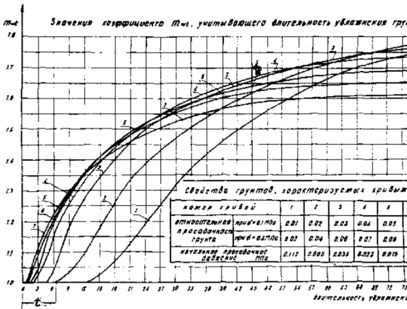
Рис. 4. Значение коэффициента m_{от} , учитывающего длительность увлажнения грунтов t
