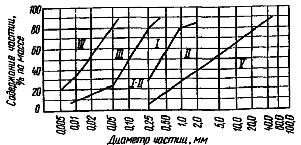
Черт. 5. Группы грунтов, используемых для намыва плотин
