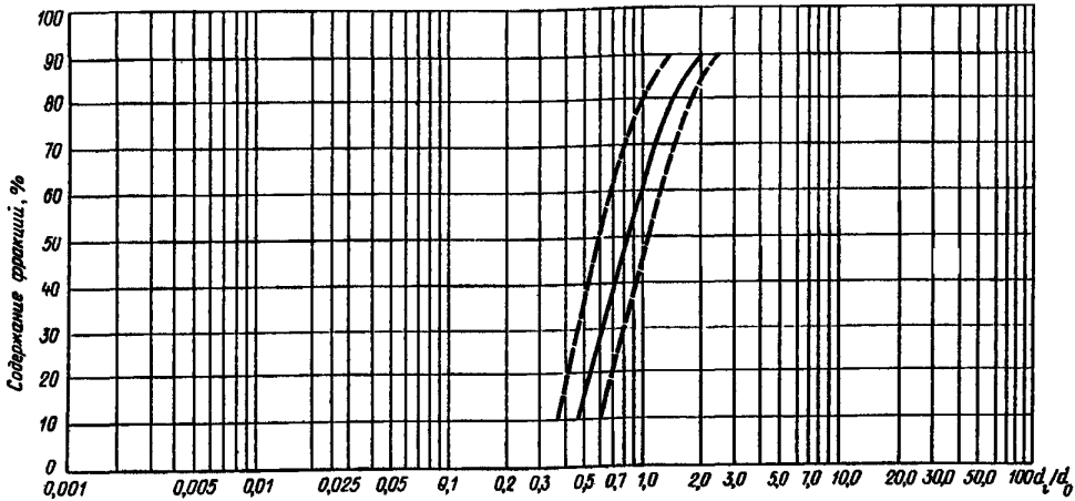
Черт. 1. График зависимости \alpha = f\left(\frac{d_i}{d_0}\right) . Однородные песчаные плотины
