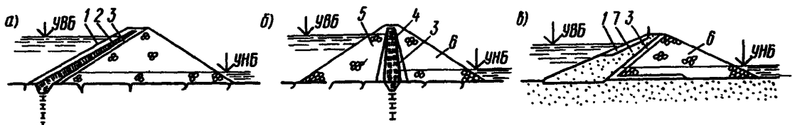
Черт. 6. Виды каменно-земляных плотин
