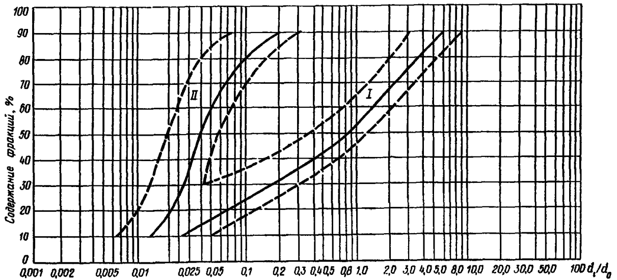
Черт. 3. График зависимости \alpha = f\left(\frac{d_i}{d_0}\right) . Неоднородные плотины из крупного песчано-гравийного грунта с центральной песчаной зоной
