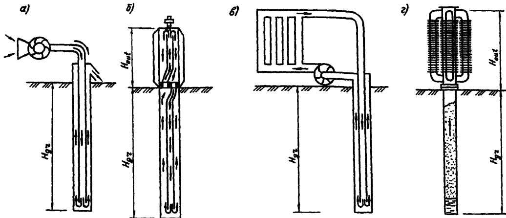
Черт. 2.1. Схемы основных видов СОУ
