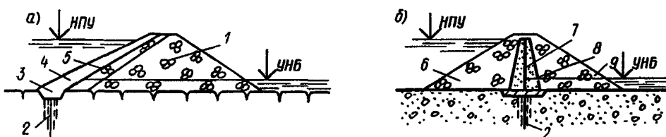
Черт. 8. Виды каменно-набросных плотин
