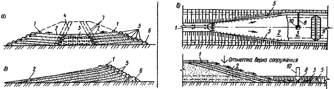
Черт. 4. Основные схемы возведения намывных плотин
