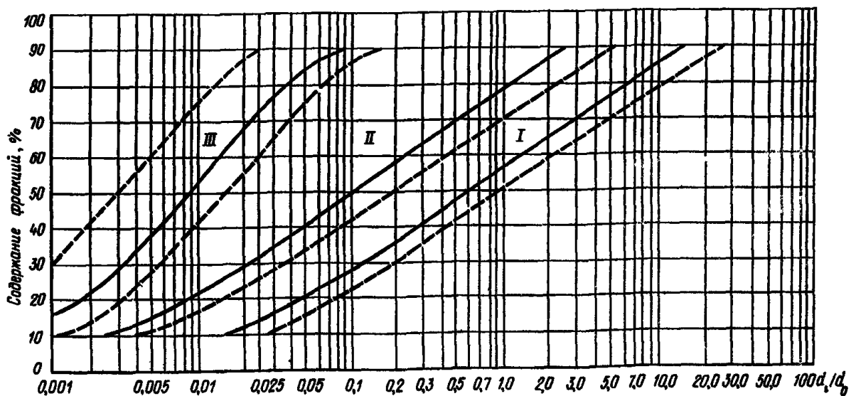
Черт. 5. График зависимости \alpha = f\left(\frac{d_i}{d_0}\right) . Гравийные плотины с ядром высотой более 30 м
