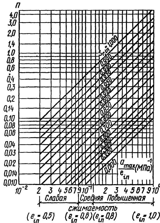
Черт. 2. Номограмма для определения параметра \Pi
