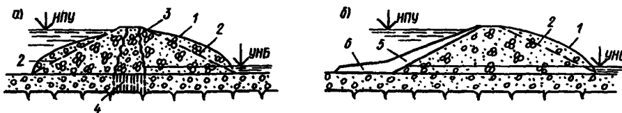
Черт. 7. Виды взрывонабросных плотин
