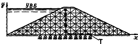
Черт. 5. Схема расчета плотины с диафрагмой по методу конечных элементов с учетом проскальзывания грунта тела плотины по основанию и диафрагме
