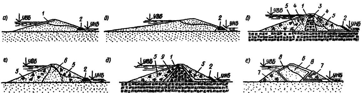
Черт. 3. Виды намывных плотин
