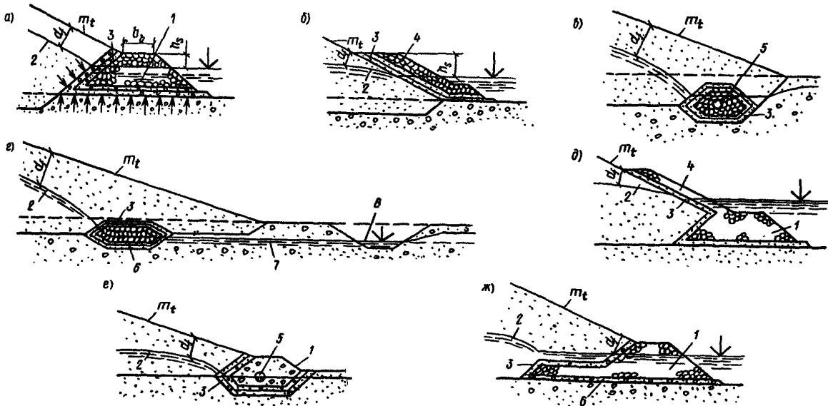
Черт. 2. Схемы основных видов дренажа
