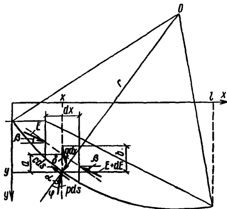
Схема сил, действующих на элемент призмы обрушения
