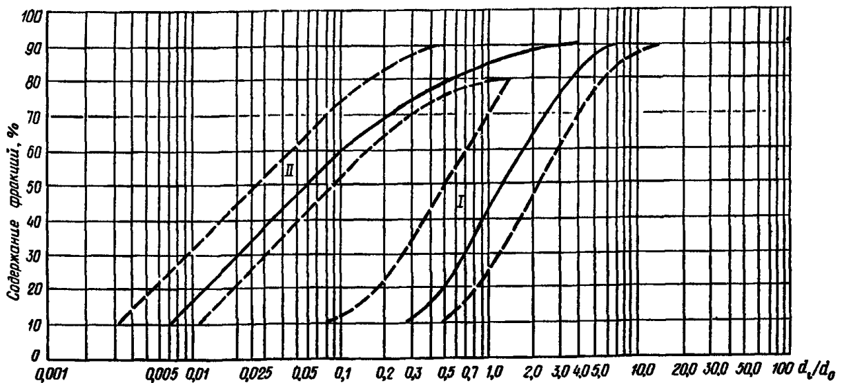
Черт. 4. График зависимости \alpha = f\left(\frac{d_i}{d_0}\right) : Гравийные плотины с ядром высотой менее 30 м
