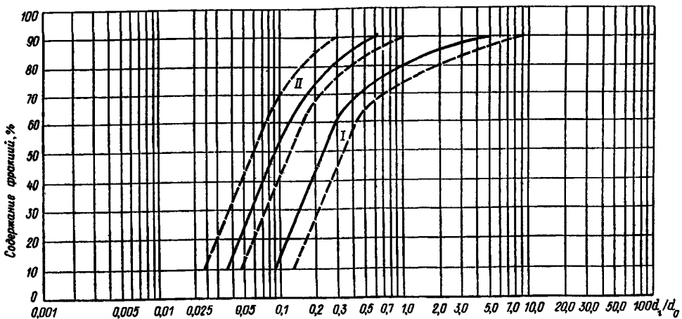
Черт. 2. График зависимости \alpha = f\left(\frac{d_i}{d_0}\right) . Неоднородные плотины из мелкого песчано-гравийного грунта с центральной песчаной зоной
