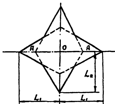
Схема обеспечения видимости на пересечениях и примыканиях
