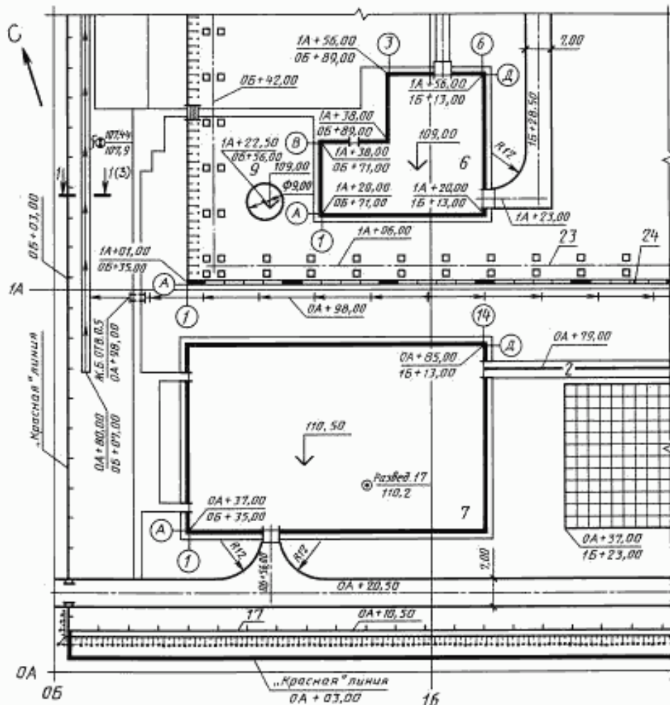
Пример оформления разбивочного плана
