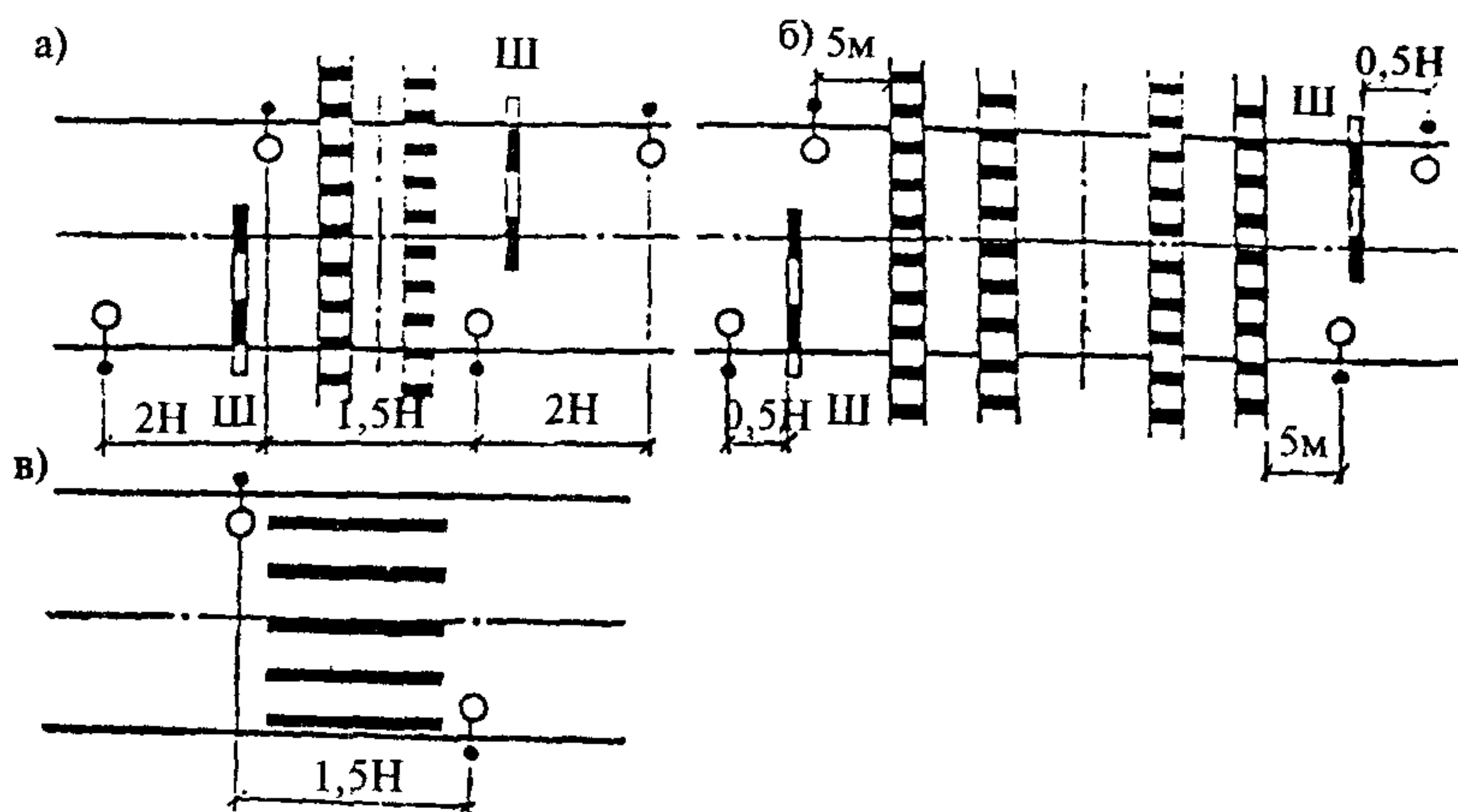
Рис. 3. Схемы размещения светильников а, б — на железнодорожных переездах; в — на пешеходном переходе; ш — автоматический шлагбаум
