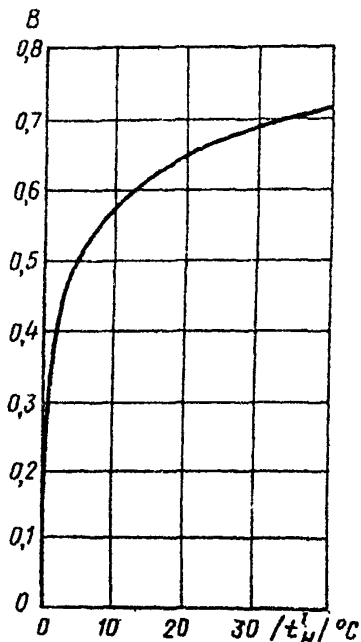
Рис. 4. Эмпирический коэффициент B для определения доли пикового догрева
