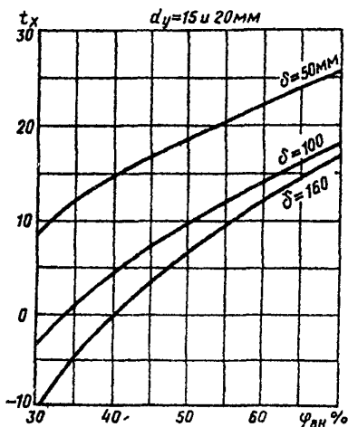
Рис. 5. Зависимость температуры хладоносителя от относительной влажности внутреннего воздуха \varphi_{вн} . d_y — условный диаметр труб, мм; \delta — толщина слоя тяжелого бетона, по нейтральной оси которого замонтированы трубы, мм.
