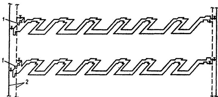
Рис. 8. Система отопления — охлаждения с дополнительными стояками 1 — задвижка на переключке, открытая зимой и закрытая летом; 2 — дополнительные стояки для режима охлаждения
