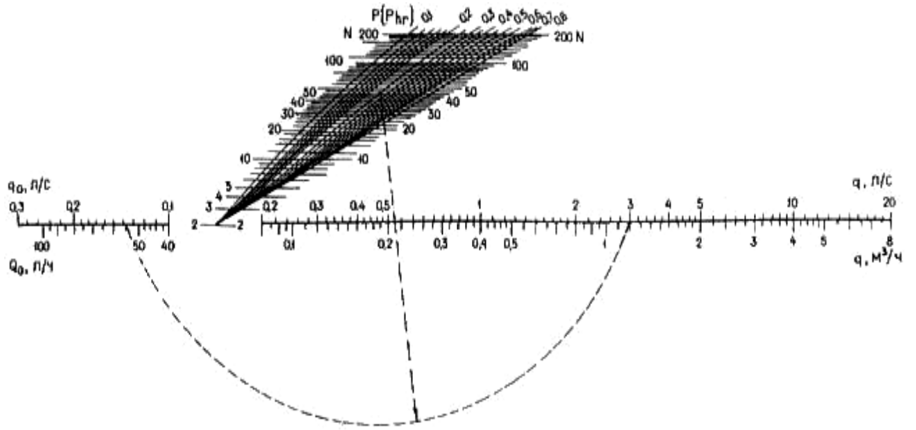
Şəkil 3. q_0 \leq 0,3 l/s, N \leq 2000 və P > 0,1 olduqda suyun saniyəlik və saatlıq sərfələrinin ( q ) təyin edilməsi üçün nomoqram
