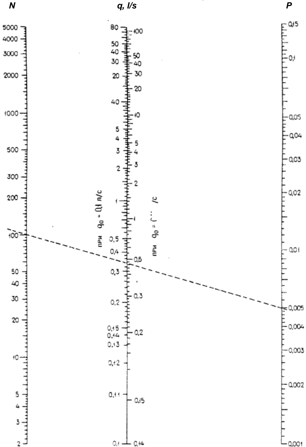
suyun saniyəlik sərfələrinin (q) təyin edilməsi üçün nomogram
