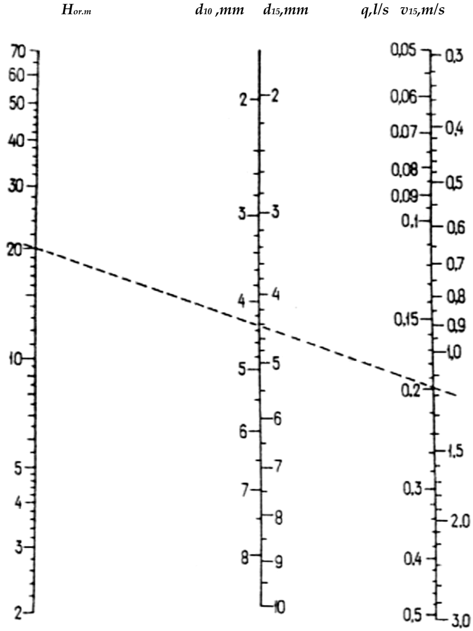
Şəkil 6. Sanitar cihazlarının qarışdırıcı armaturunda qoyulan diafraqmaların deşiklərinin diametrlərini təyin etmək üçün nomogram d_{10} ( d_{15} ) - şərti keçid diametri d = 10 və 15 mm olan qarışdırıcı armaturun birləşdirici borularında qoyulan diafraqmanın deşiyinin diametri; v_{15} - diametri 15 mm olan boruda suyun hərəkət sürətidir, m/s .
