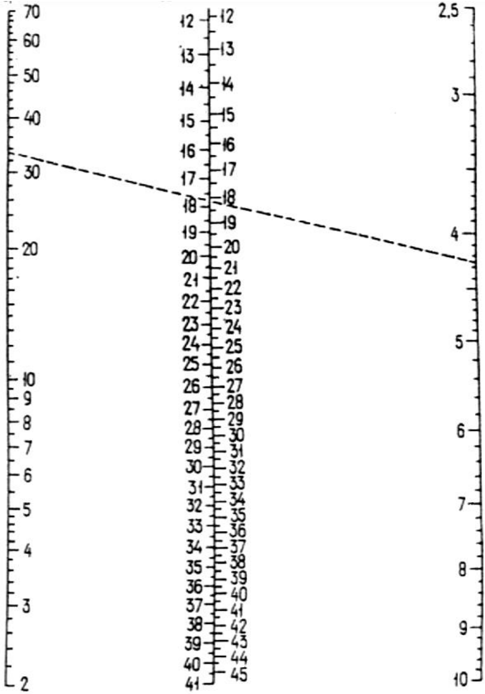
Şekil 5. Birləşdirici başlıqlar və yağın kranları arasında qoyulan diafraqmaların deşiklərinin diametrlərini təyin etmək üçün nomogram
