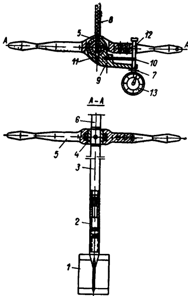
Рис. 23. Сдвигомер-крыльчатка СК-8
