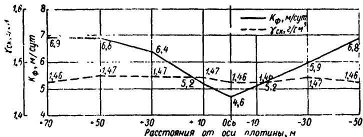
Рис. 9. График изменения объемного веса скелета намытого грунта и коэффициента фильтрации в пределах яруса сооружения (для сдвонной плотины).
