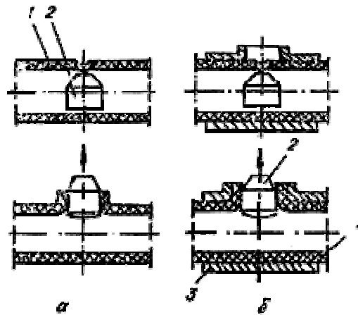
Рис.3. Схема процесса вытяжки горловин в трубах: а - при помощи пуансона (без формирования толщины стенок горловины); б - при помощи пуансона и матрицы (с формированием толщины стенок горловины); 1 - труба с отверстием; 2 - пуансон; 3 - матрица
