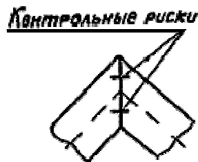
Рис.12. Расположение контрольных рисок на трубах при ручной сварке
