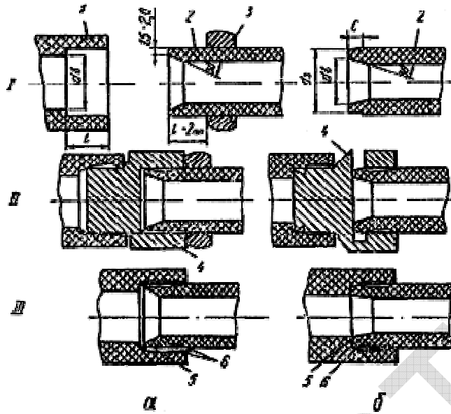
Рис.7. Последовательность процесса контактной сварки труб:
