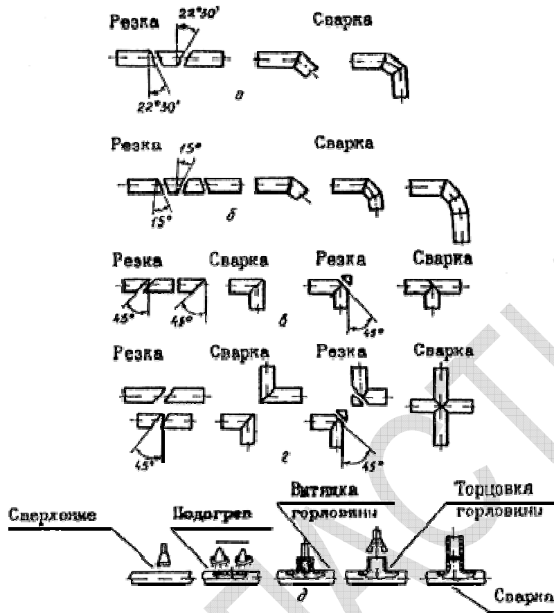
Рис.11. Схема процесса изготовления соединительных деталей при помощи контактно-стыковой сварки: а - односекторных отводов; б - двухсекторных отводов, в - тройники равнопроходных; г - крестовин; д - тройники переходных
