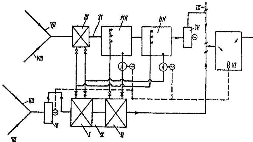
Рис. 7. Принципиальная схема двухпозиционного регулирования бескомпрессорной системы кондиционирования воздуха
