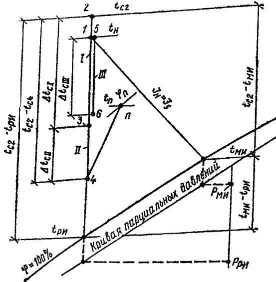
Рис. 12. Графическая интерпретация расчетных зависимостей при работе испарительного кондиционера на наружном воздухе
