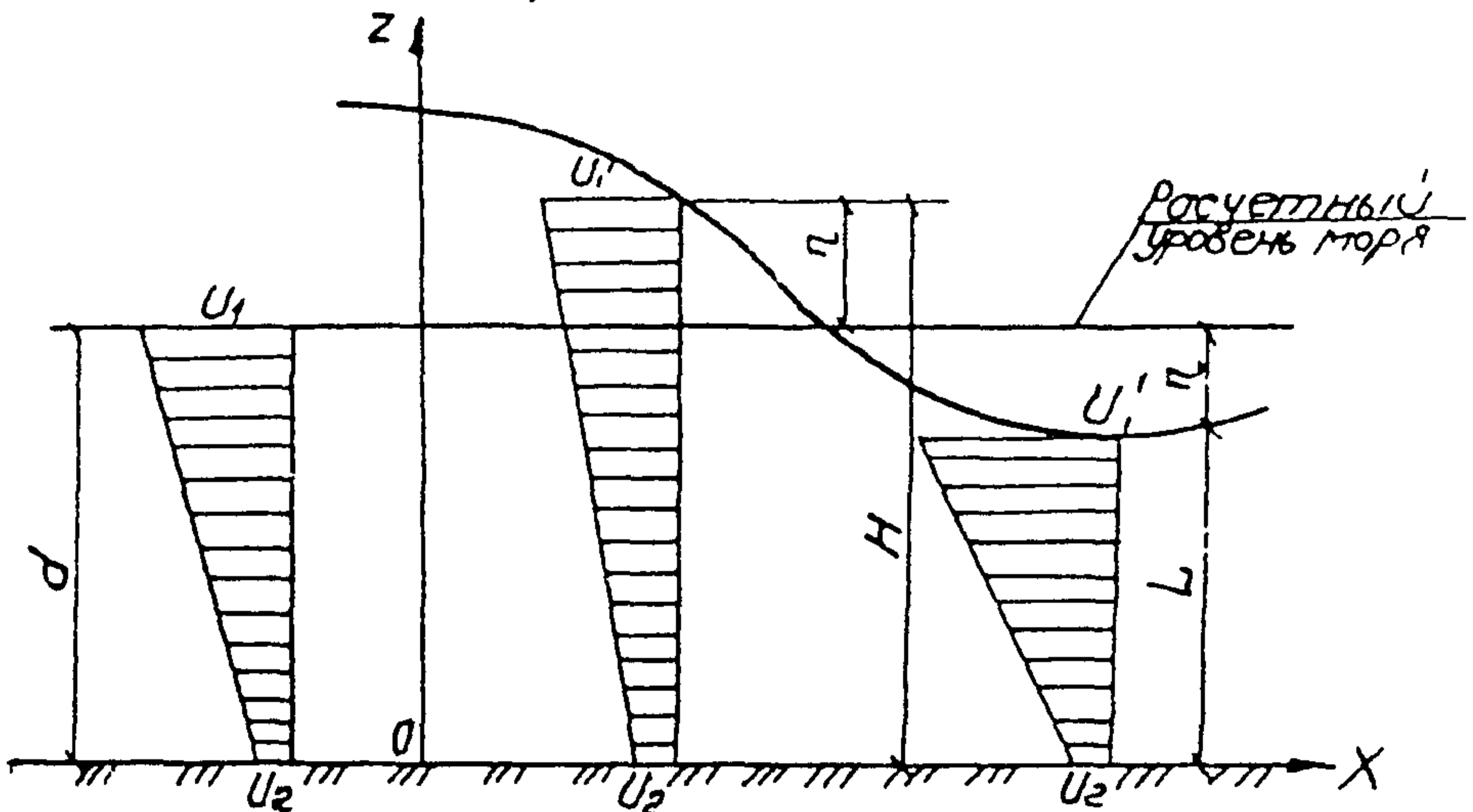
Эпюры скорости течения при различных фазах волны
