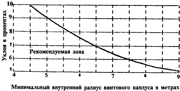
График 2. Зависимость внутреннего радиуса винтового пандуса от величины его уклона
