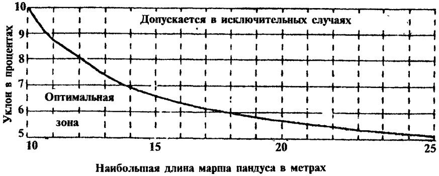
График 1. Зависимость длины марша пандуса от величины его уклона
